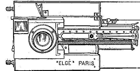
FIG. 10 bis. — Chambre à main pour contrôle de la vitesse des automobiles.
